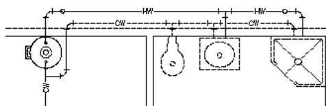
Résultat de la connexion de la ligne de plomberie sélectionnée aux appareils sanitaires
