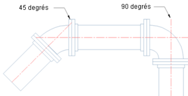
Trait d'axe d'un tuyau en affichage 2D
